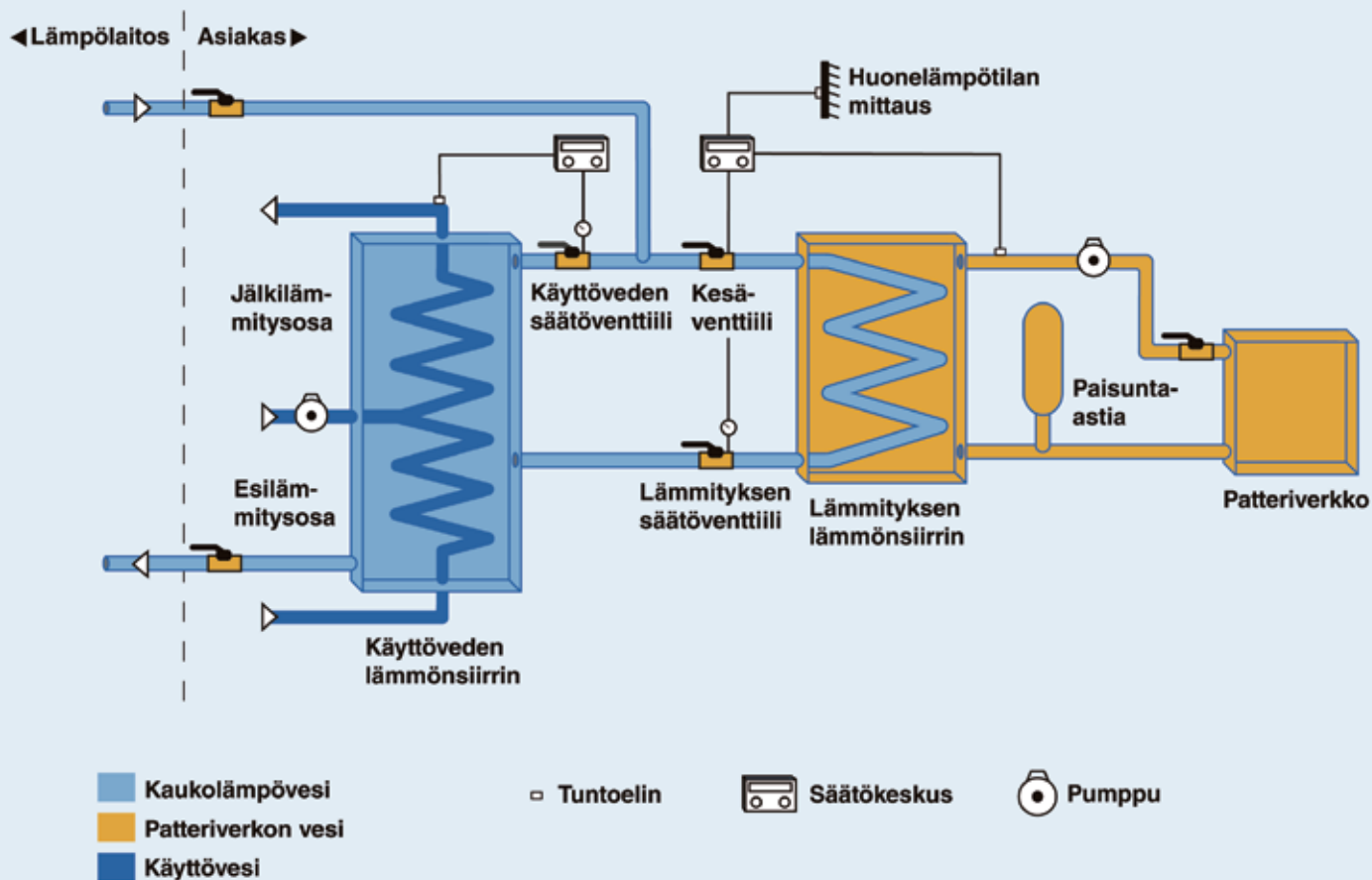
Kaaviokuva kaukolämmön toimintaperiaatteesta. Katkoviivasta oikealla olevat laitteet ovat asiakkaan vastuulla.
